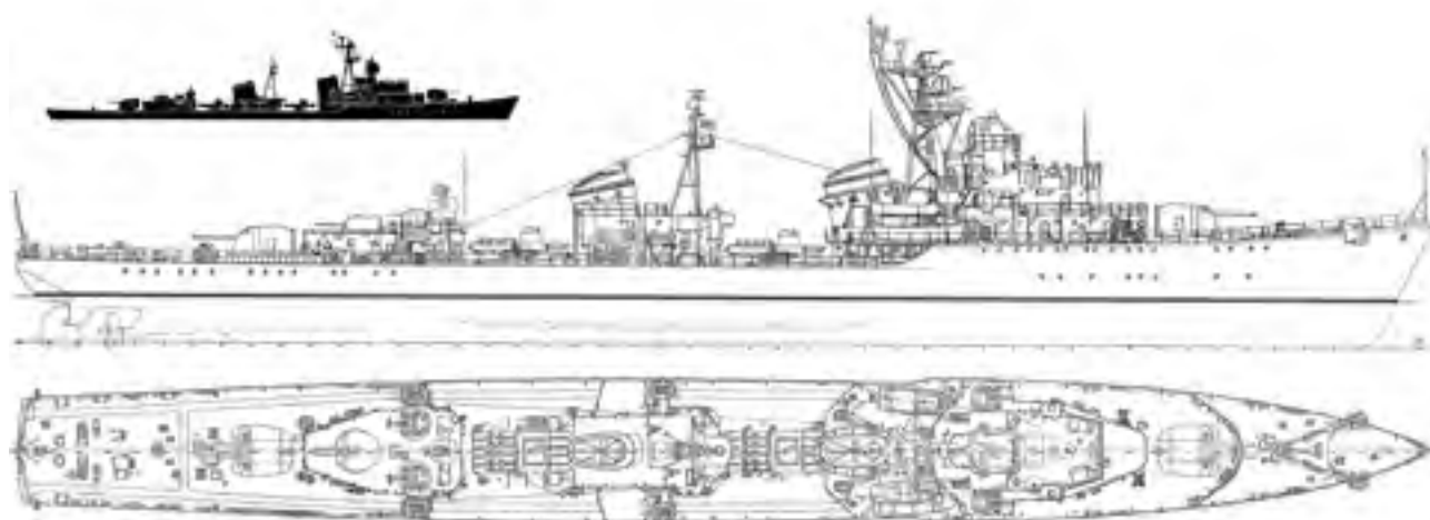
ЭСКАДРЕННЫЙ МИНОНОСЕЦ пр. 30бис
